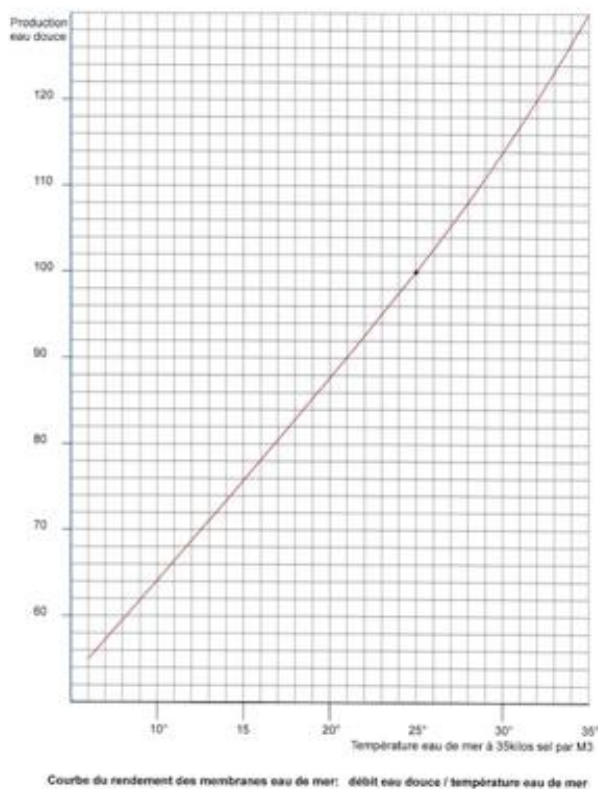
Courbe du rendement des membranes eau de mer: débit eau douce / température eau de mer
